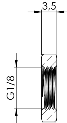
SCHNITT A-A
