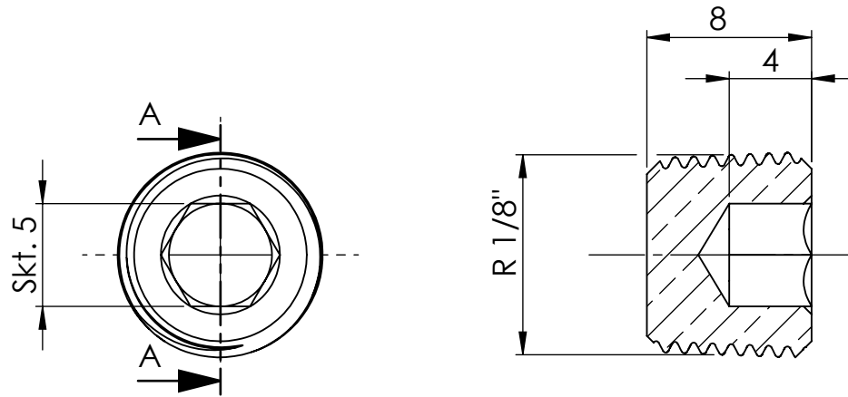
Ansicht / view A-A
