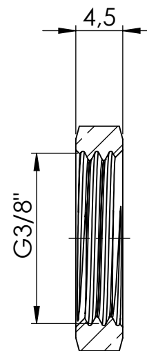
Ansicht / view A-A
