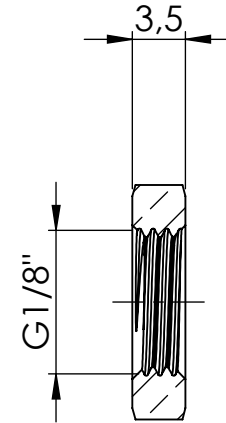
Ansicht / view A-A
